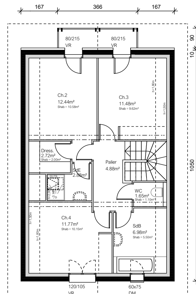
Plan Etage
